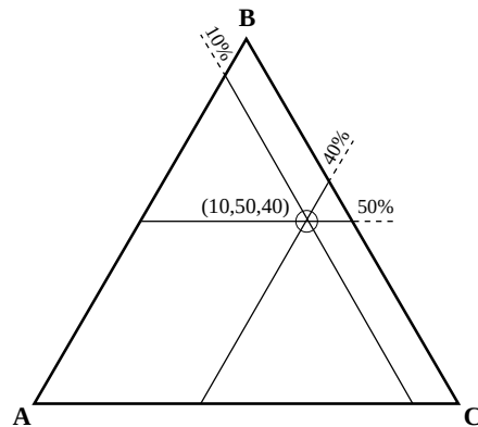
Gambar 7.4.: Prinsip pengeplotan diagram segitiga
