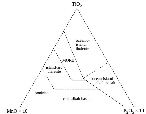
Gambar 7.5.: Contoh penerapan diagram segitiga
