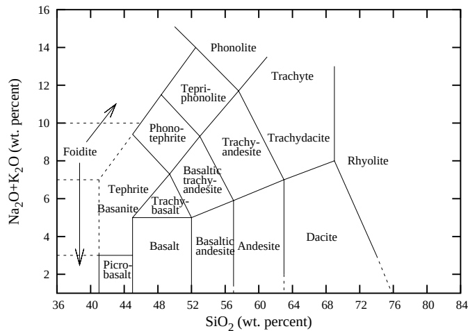
Gambar 7.1.: Klasifikasi batuan dengan diagram TAS
