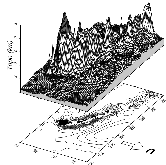
Gambar 8.4.: Contoh pengkonturan dan tampilan 3-D dengan GMT
