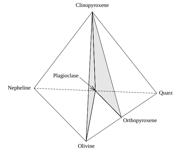
Gambar 7.7.: Contoh penggunaan diagram piramida dalam geologi
