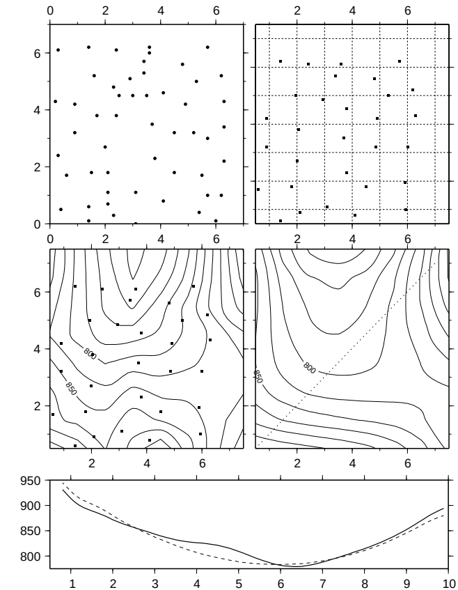
Gambar 8.5.: Contoh pengkonturan dan pembuatan penampang
