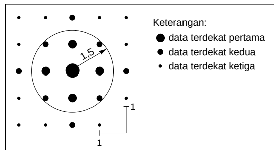
Gambar 8.6.: Data yang telah diubah dalam bentuk diskret
