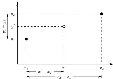
Gambar 3.1.: Interpolasi linear antara dua titik data
