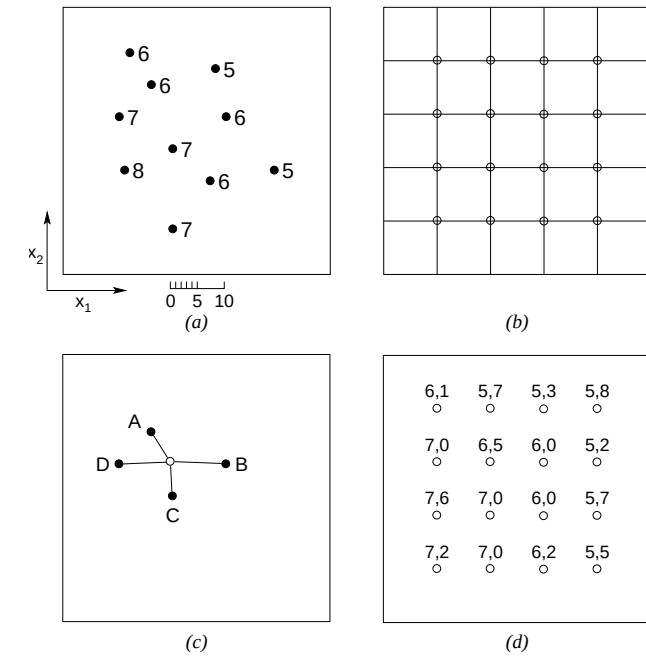
Gambar 8.2.: Langkah-langkah dalam perhitungan nilai diskret dari data acak. (a) titik-titik yang tersebar secara acak. (b) jaring-jaring diskret dengan notkah diskret yang akan dihitung. (c) lokasi 4 buah titik kontrol terdekat untuk sebuah titik diskret. (d) titik diskret yang telah dihitung lengkap (Davis, 1986, 2002).
