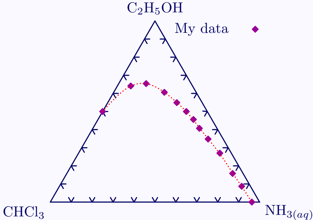
Gambar 1: Diagram segitiga yang dibuat dengan gnuplot
